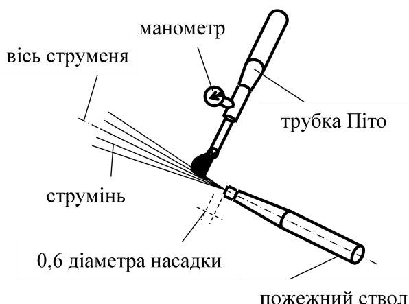
Рисунок 8.6 – Використання трубки Піто для визначення кількості води
