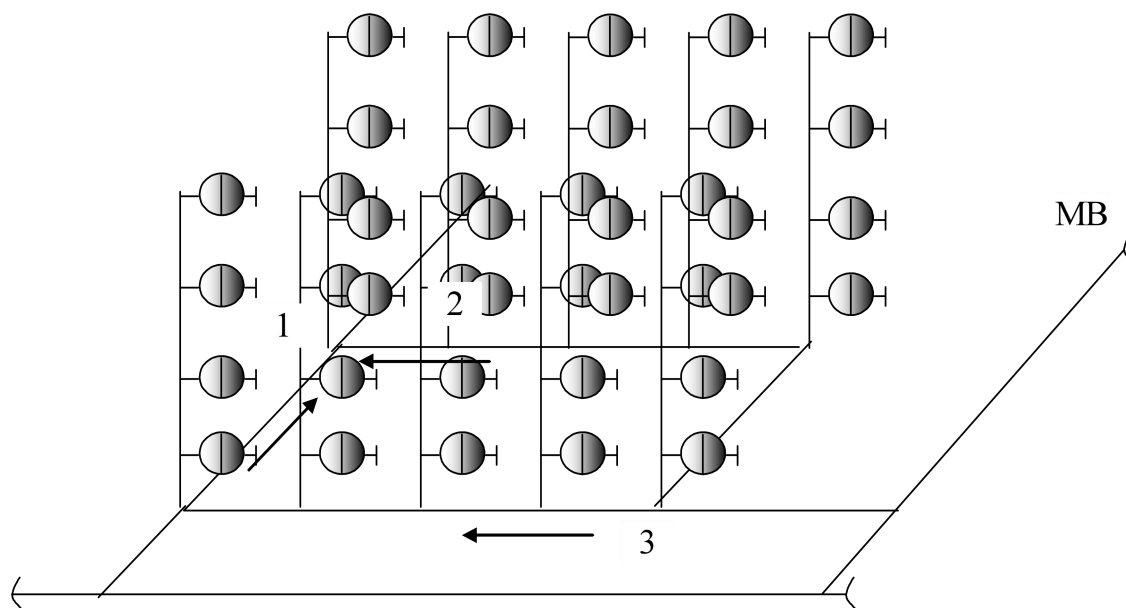
Рисунок 5.2 – Приклад побудування аксонометричної схеми ВВП будівлі та підготовки її до розрахунку
