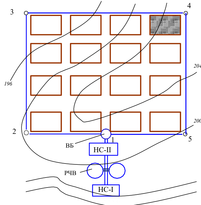
Рис. 1.1 – Трасування водопровідної мережі населеного пункту
