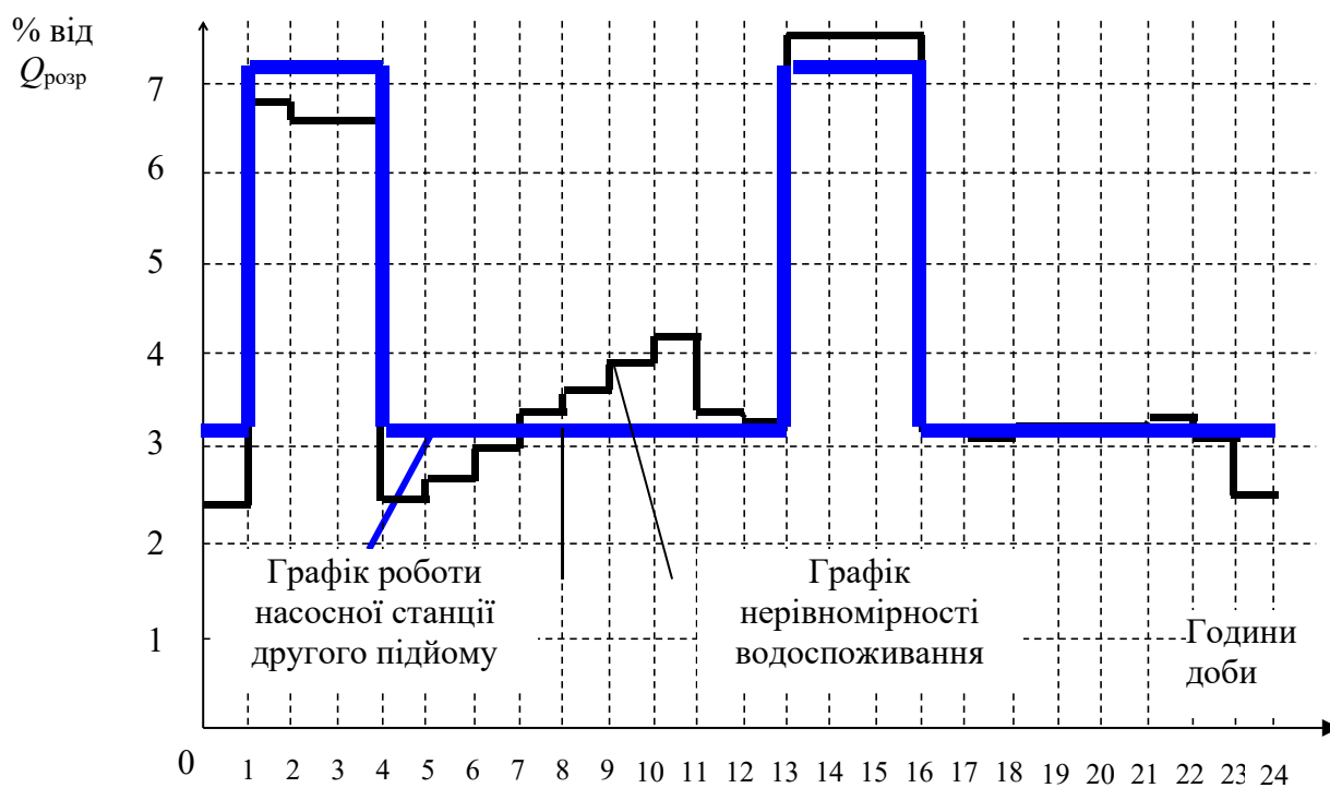
Рис. 4.1 – Графіки нерівномірності водоспоживання та режиму роботи насосної станції II підйому
