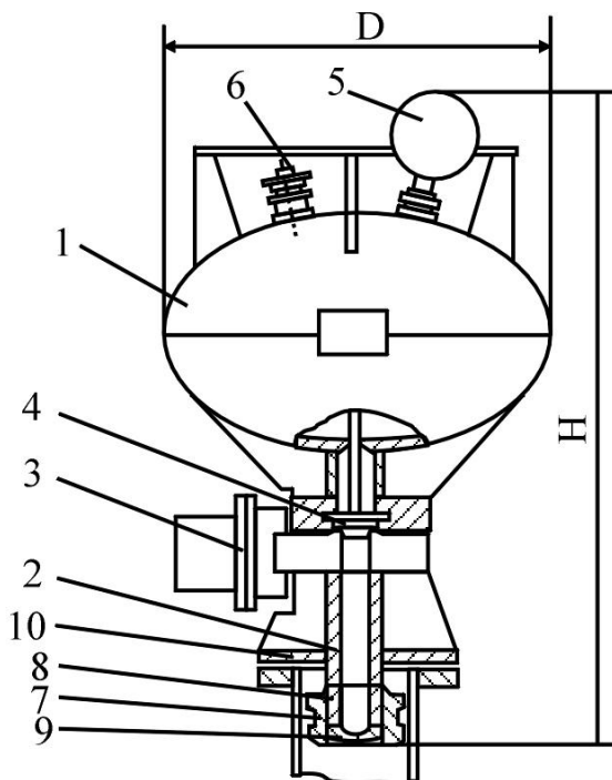
Рис. 4.7 – Зрошувач:
