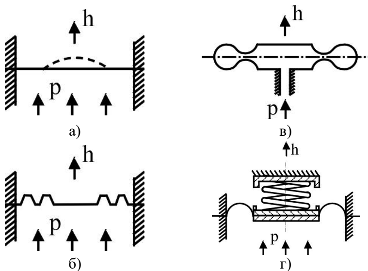
Рис. 2.44 – Мембранні чутливі елементи:
