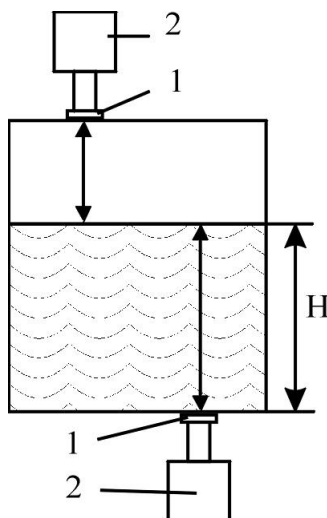
Рис. 2.64 – Ультразвуковий і акустичний рівнеміри:
