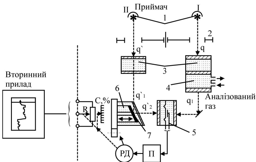
Рис. 2.80 — Схема автоматичного оптико-акустичного газоаналізатора типу ОА
