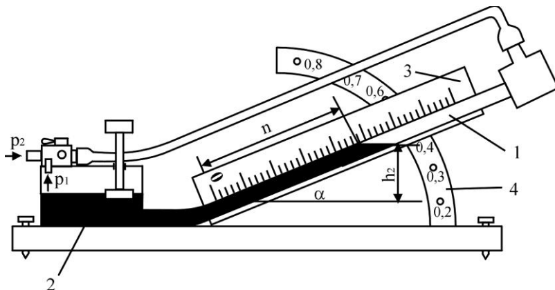
Рис. 2.34 – Схема мікроманометра: 1 – складова трубка; 2 – резервуар з рідиною; 3 – шкала; 4 – нахилений упор.
