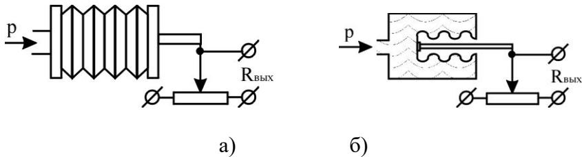
Рис. 2.42 – Датчики тиску:
