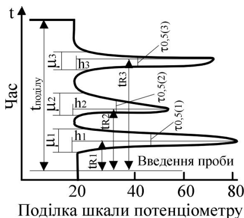
Рис. 2.82 – Хромотограма поділу суміші трьох компонентів
