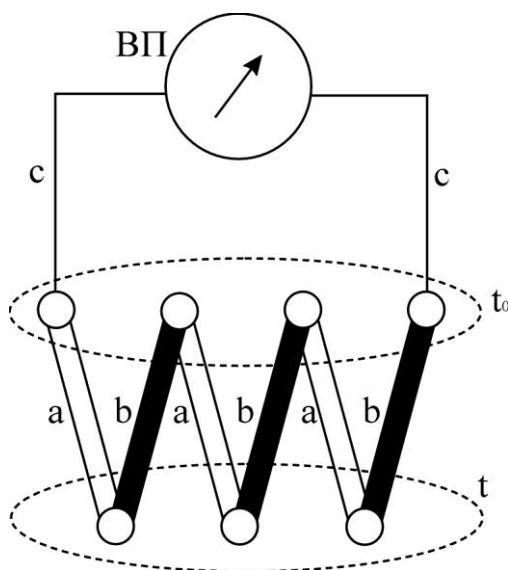
Рис. 2.10 – Термобатарея
