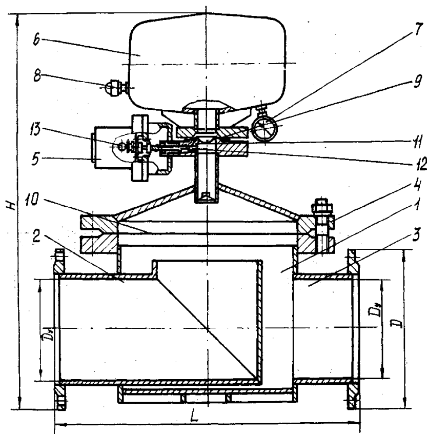
Рис. 4.9 – Полум'явідсікач ПО-1Ш:
