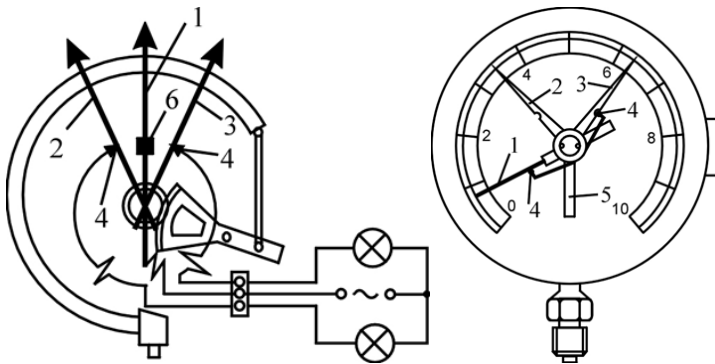
Рис. 2.38 – Електроконтактний манометр
