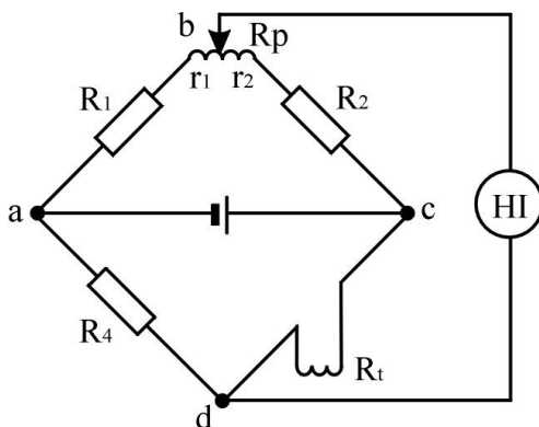
Рис. 3.2 – Вимірювальний міст:
