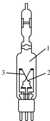
Рис. 2.52 – Термопарний манометричний перетворювач
