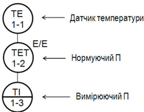
Рис. 7.4 – Приклад функціональної групи приладів вимірювання температури
