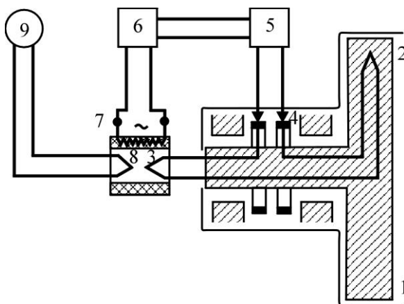
Рис. 2.24 – Схема виміру температури обертювх деталей термоелектричним термометром
