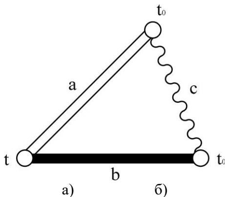
Рис. 2.7 – Включення третього провідника в ланцюг термопар
