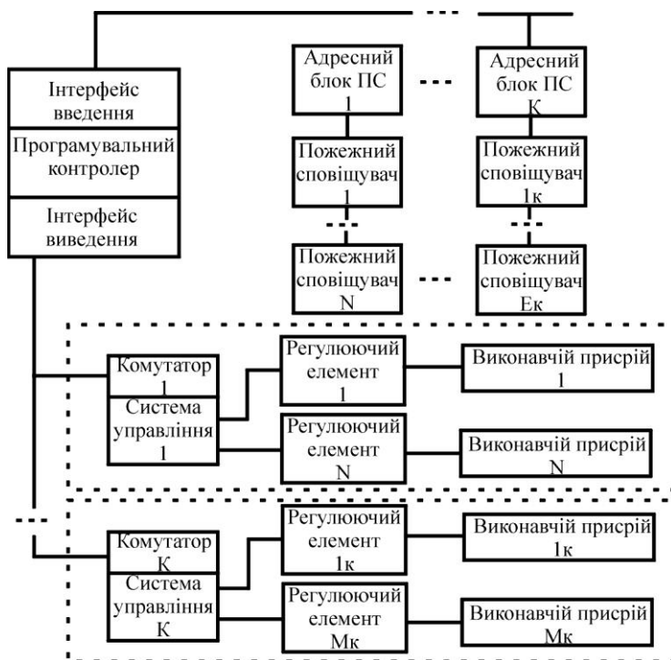
Рис. 1.5 – Структурна схема ЛАСППЗ із комутаторами
