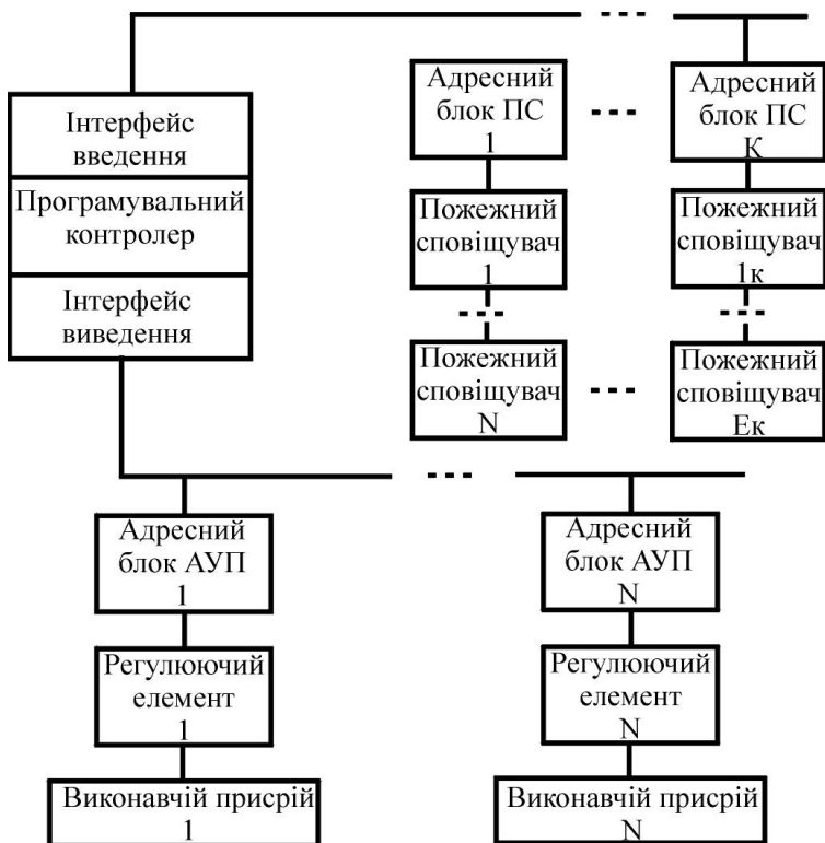
Рис. 1.4 – Структурна схема ЛАСПЗ з адресними блоками
