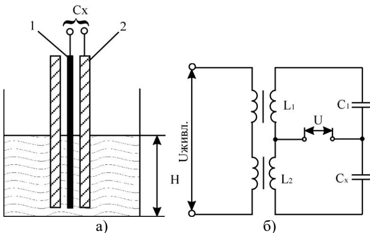
Рис. 2.59 – Ємнісний рівнемір:
