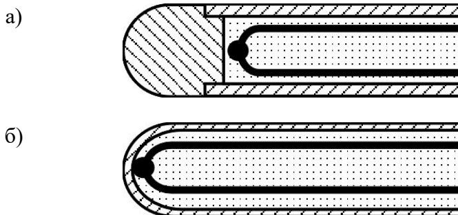
Рис. 2.12 – Будова термометрів кабельного типу:
