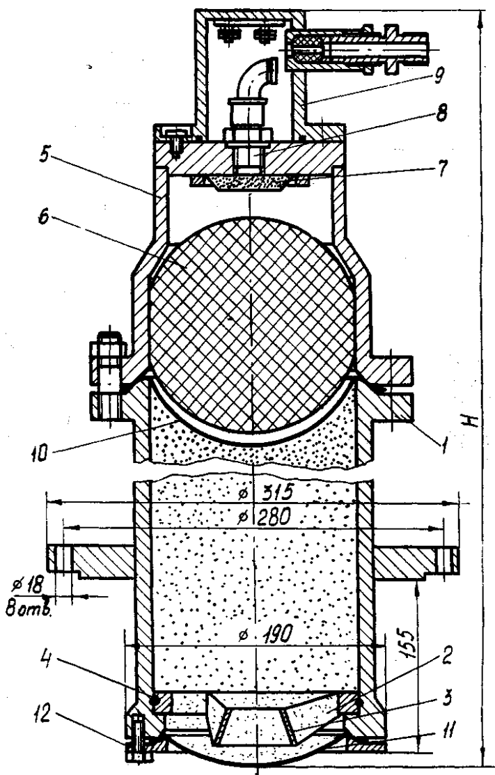
Рис. 4.6 – Порошковий полум'япридушувач:
