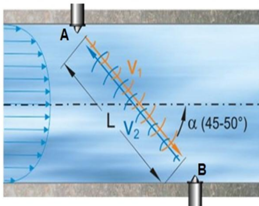
Рис. 2.71 – Схема ультразвукового витратоміра
