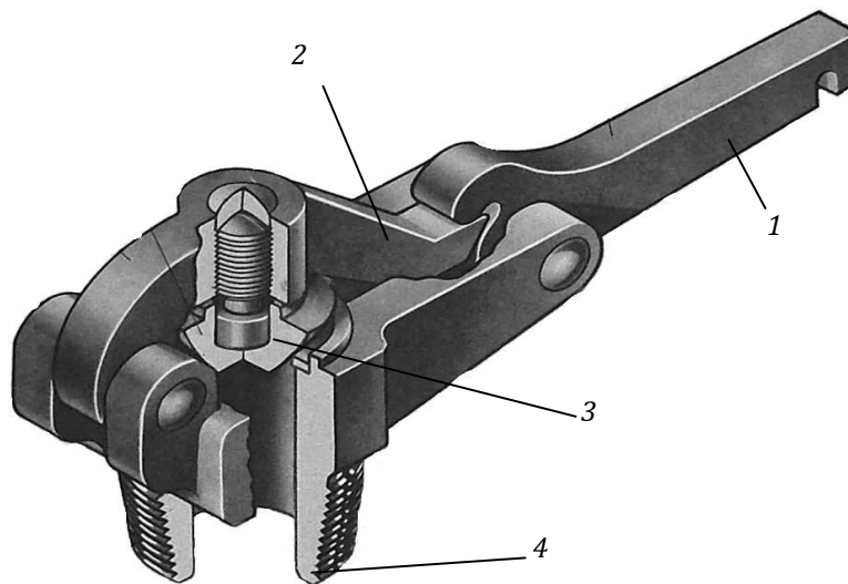
Рис 1.13 – Спонукальний клапан:
