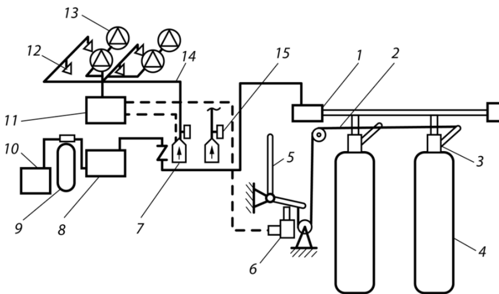
Рис. 2.28 – Установка газового пожежогасіння з електричним пуском УАГЕ:
