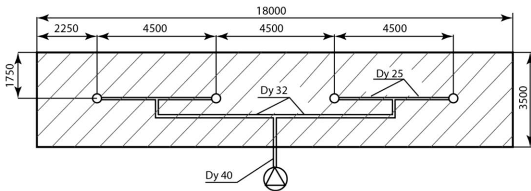
Рис. 3.36 - Трубна розводка
