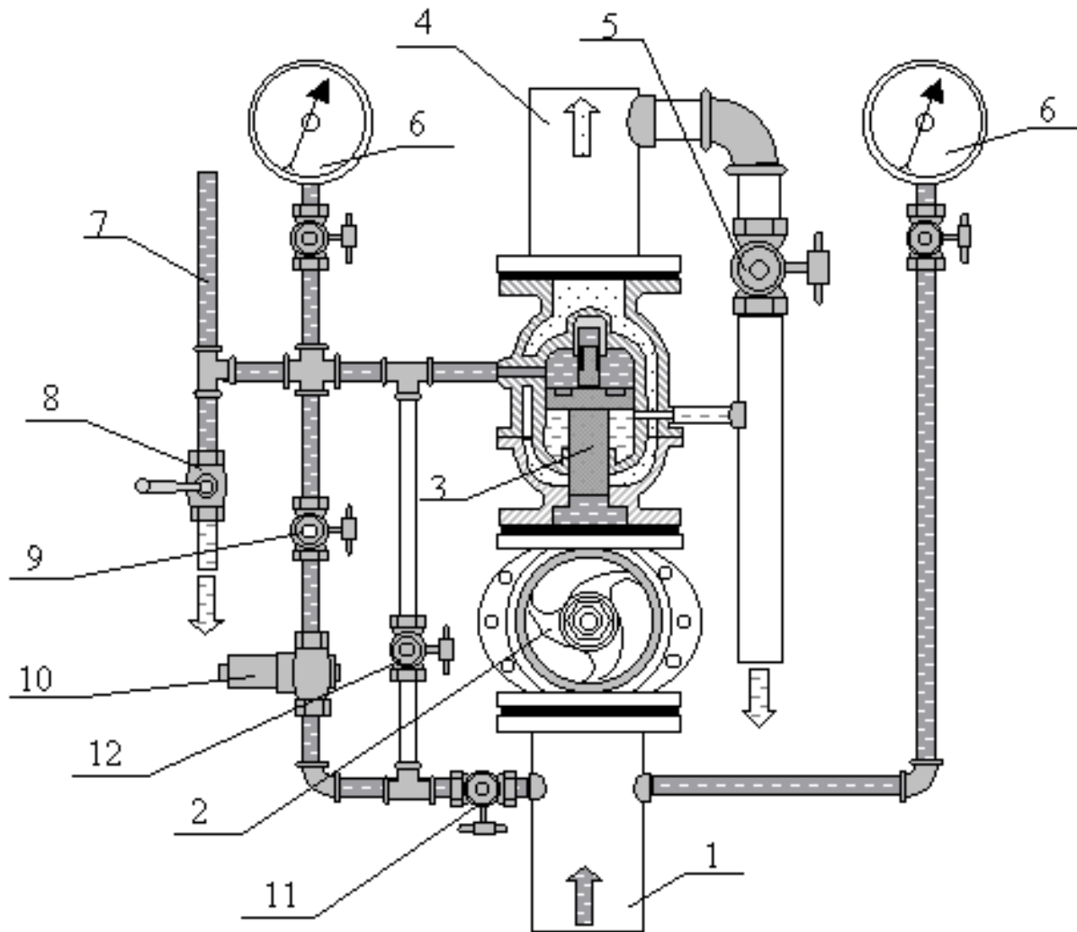
Рис. 1.19 – Вузол керування дренчерної системи зі швиглядкодіючим клапаном:
