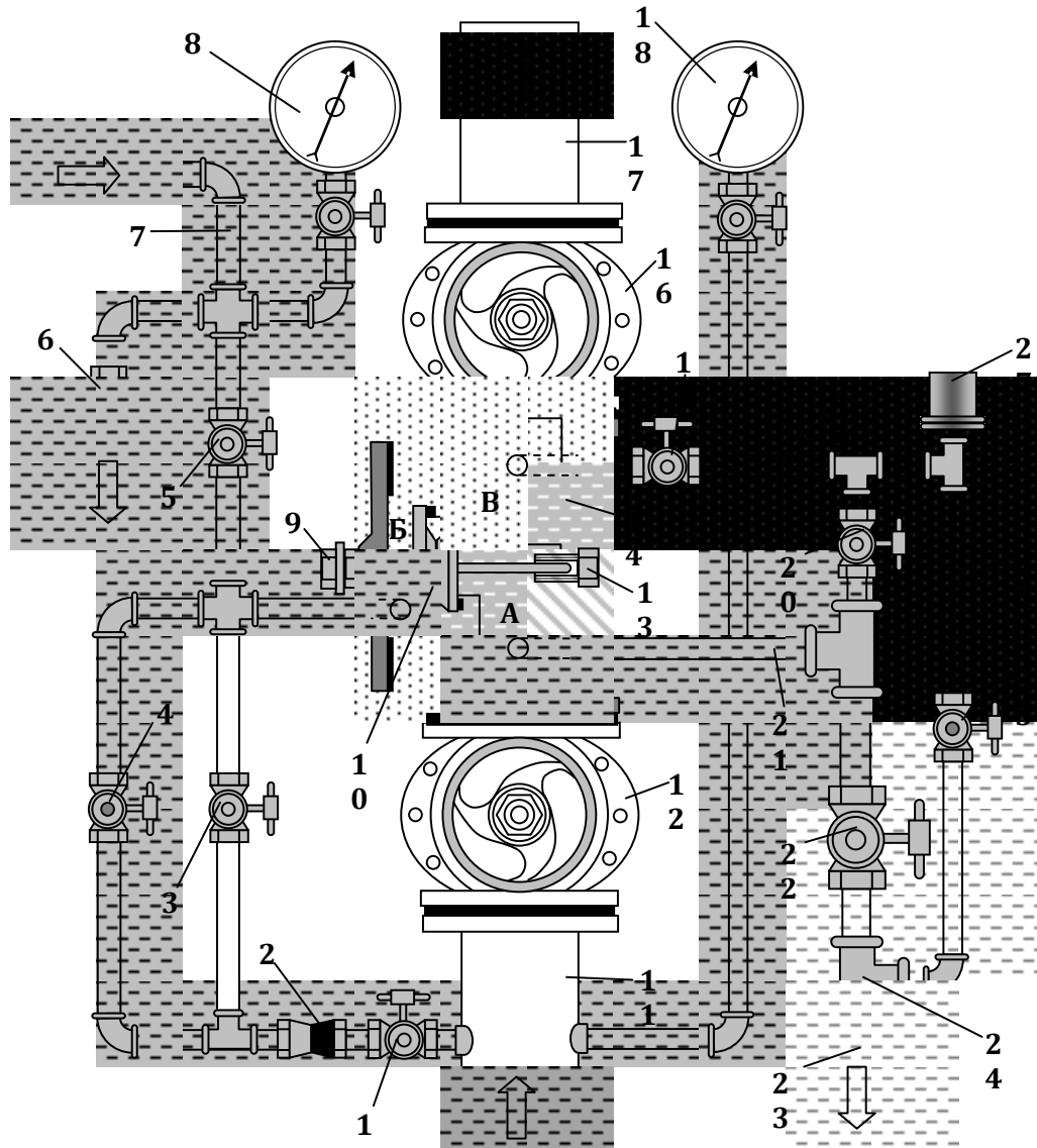
Рис. 1.17– Вузол керування автоматичної дренчерної системи із клапаном групової дії
