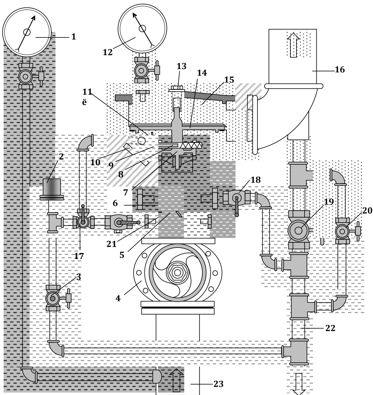
Рис. 1.16 – Вузол керування повітряний водяної спринклерної системи із клапанами В і ВС:
