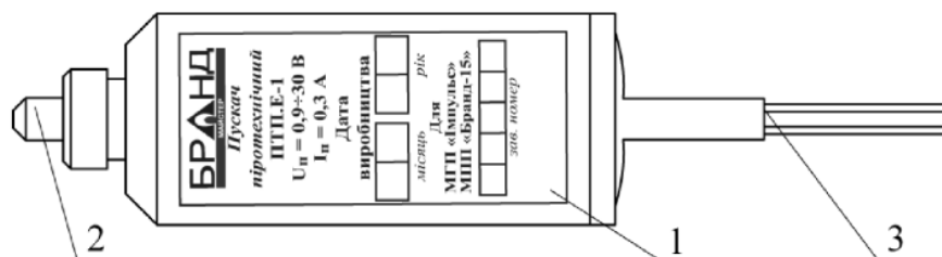
Рис. 2.8 – Піротехнічний пускач:
