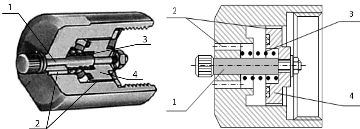
Рис. 2.23 – Секційний запобіжник:
