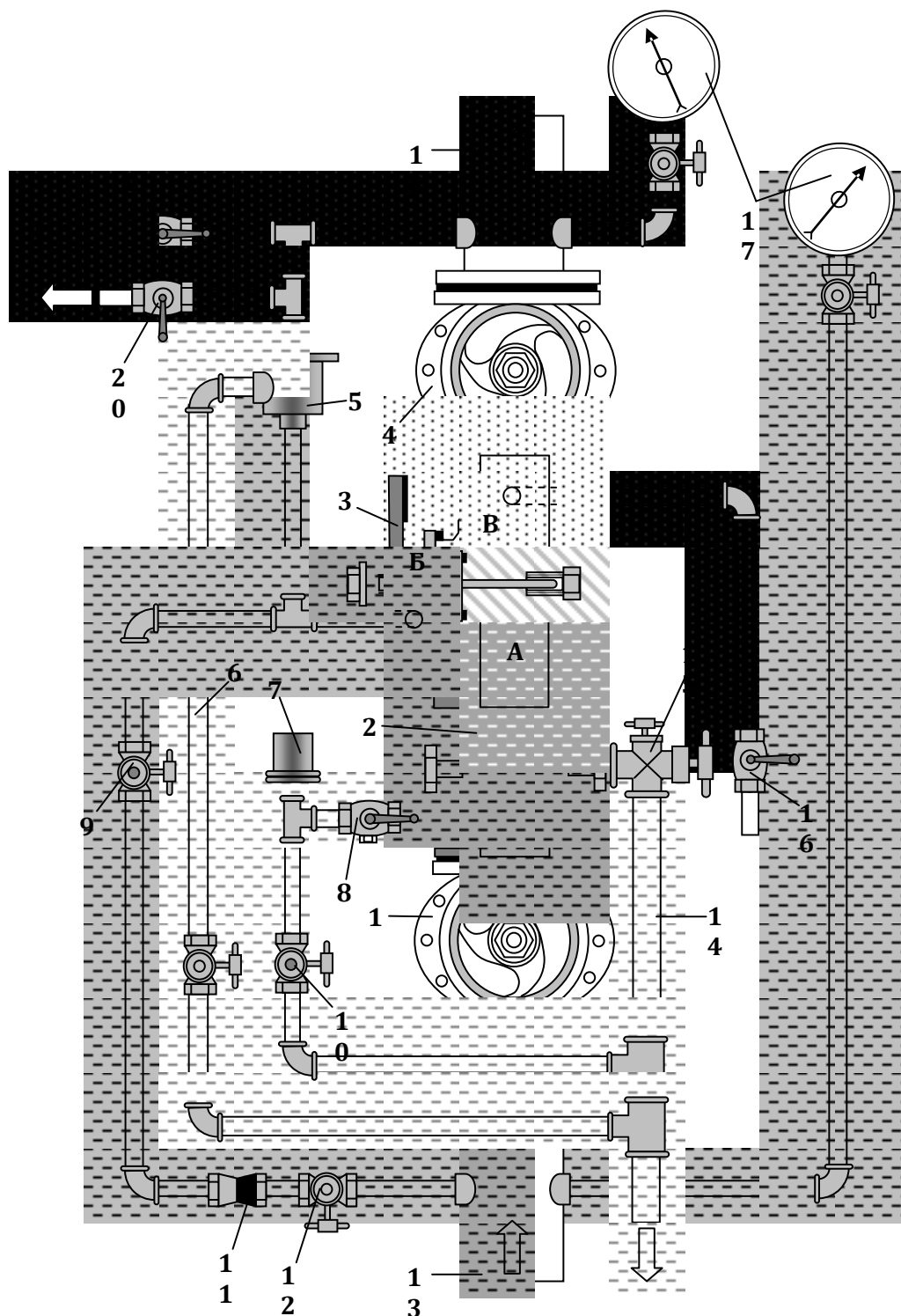
Рис. 1.18 – Вузол керування повітряно-водної спринклерної системи із клаванами ВС, ГД, КПВ:
