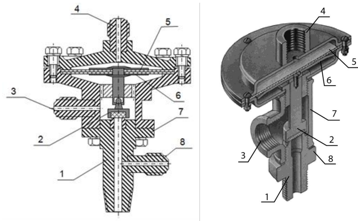
Рис. 2.24 – Клапан пусковий повітряний КПВ:
