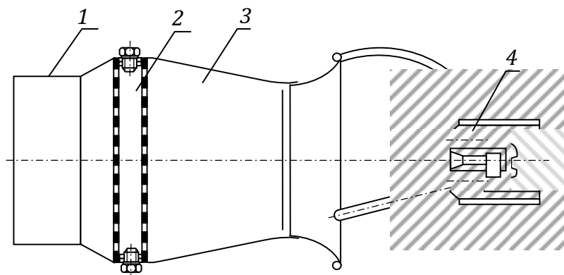
Рис. 1.25 – Генератор повітряно-механічної піни середньої кратності для стаціонарної системи типу ГПСС:
