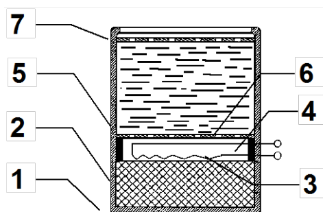
Рис. 4.12 – Конструкція генератора МАГ з насипним теплопоглиначем:
