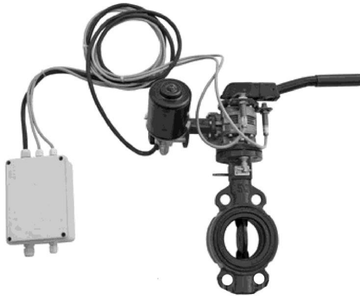
Рис. 1.46 – Дискові затвори з електроприводом Ду80 (12;24 В)
