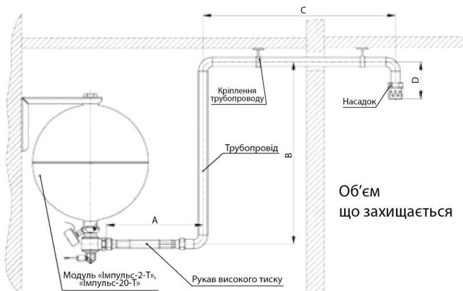
Рис. 2.13 – Умовна схема монтажу модуля з використанням трубопроводу
