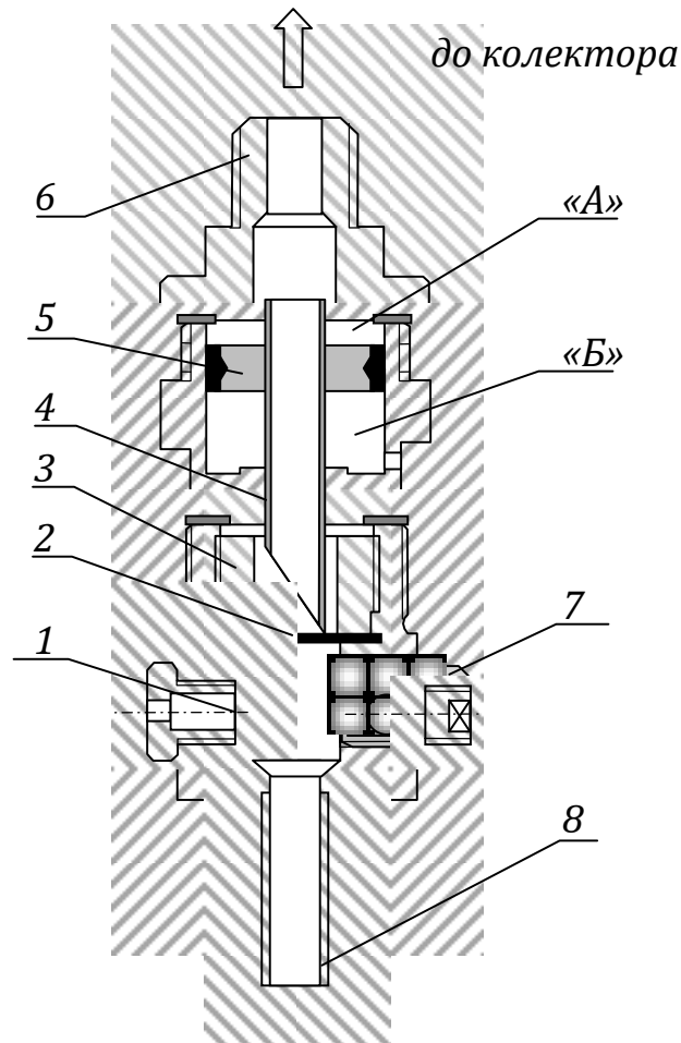
Рис. 2.1 – Головка випуску заряду ГАВЗ:
