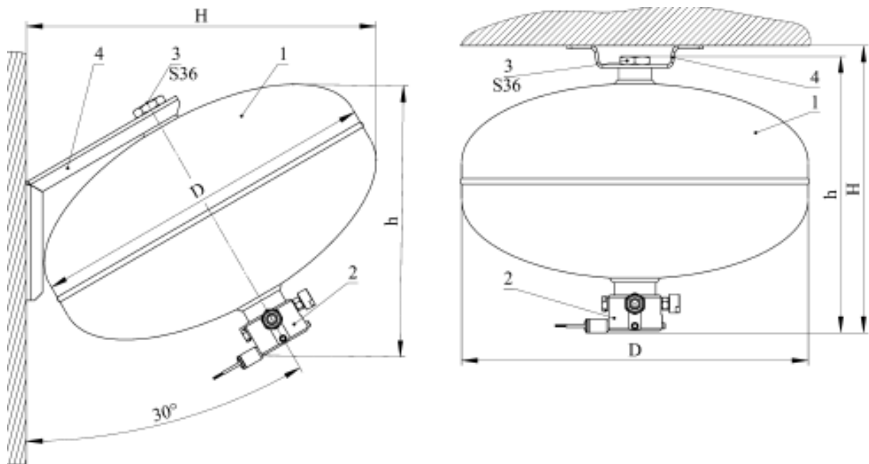
Рис. 3.29 – Загальний вигляд МПП «БРАНД»:
