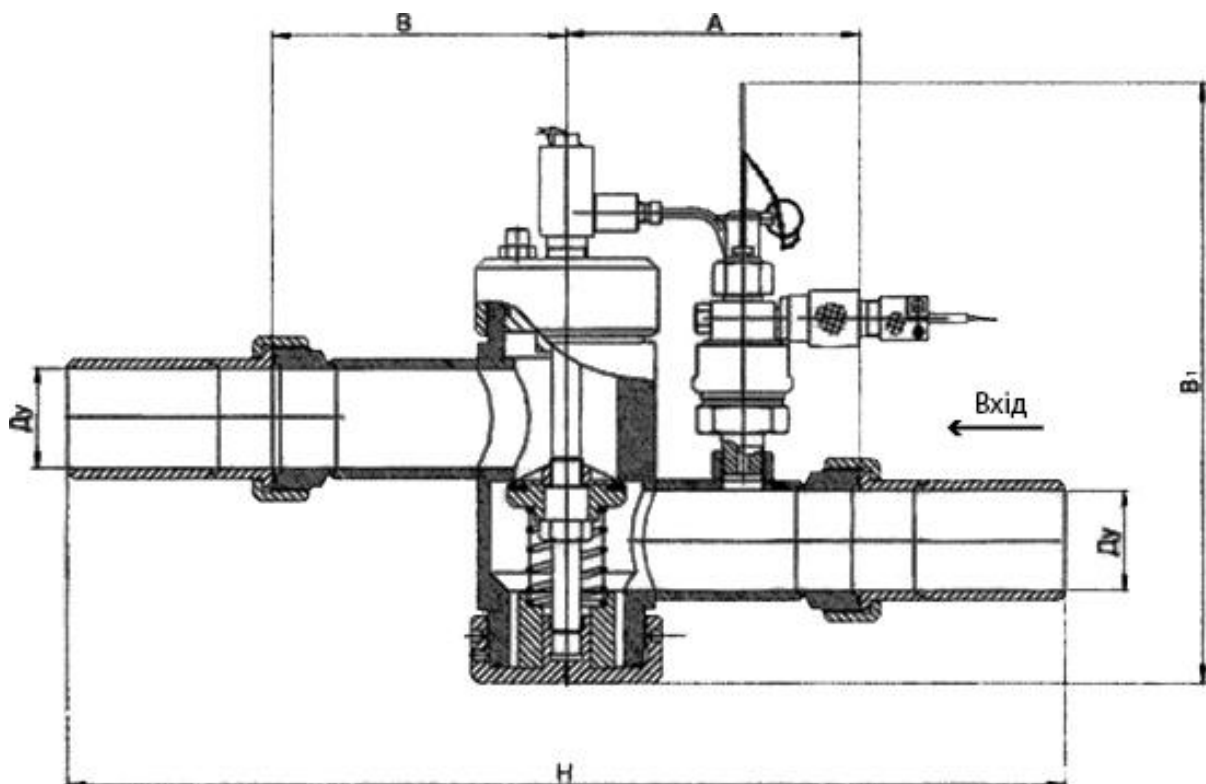
Рис. 2.19 – Конструкція розподільчого пристрою РУ МЕЗ (1М) -50 (80)
