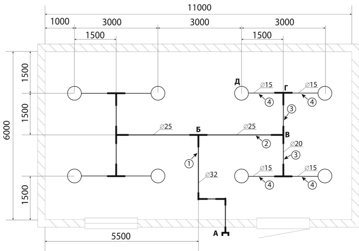
Рис. 2.32 – Збалансована розподільча мережа АСП високого тиску для захисту приміщення
