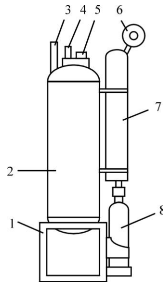
Рис. 3.2 – Загальний вигляд порошкового вогнегасника типу ОПА:
