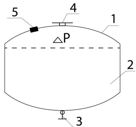
Рис. 3.28 – Принципова схема модуля порошкового пожежогасіння «Пума-12П»:
