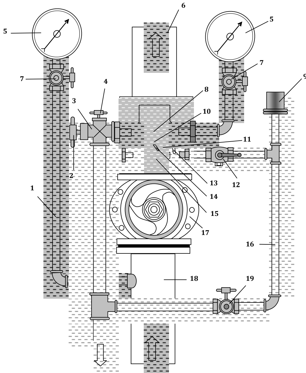
Рис.1.14 – Вузол керування спринклерної системи із клапаном ВС:
