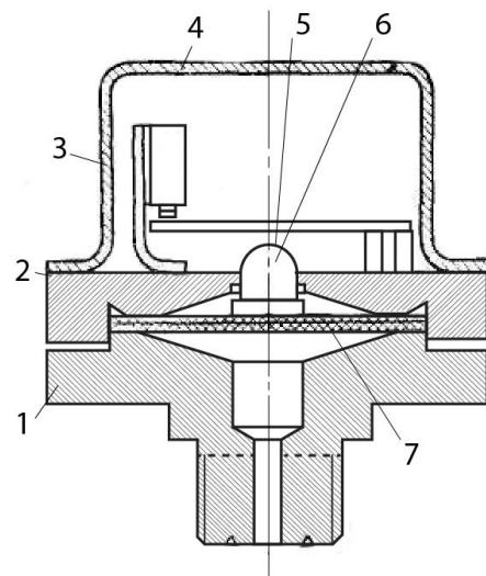
Рис 1.5 – Конструкція сигналізатора тиску універсального:
