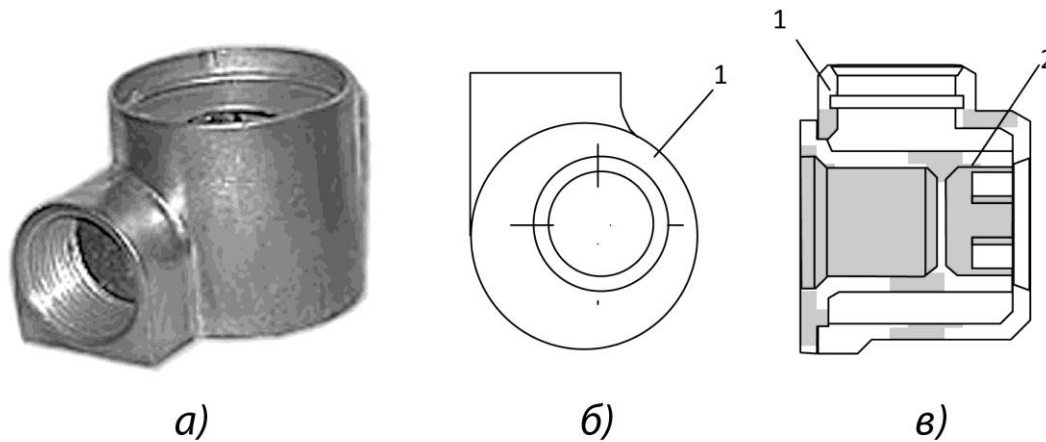
Рис 1.24 – Зрошувач евольвентний:
