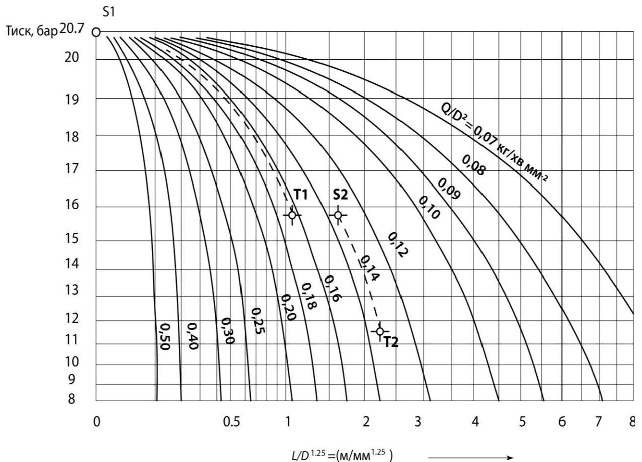
Рис. 2.34 – Падіння тиску у трубопроводі за умови, що тиск у резервуарі становить 20,7 бар
