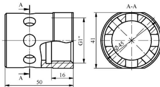
Рис. 2.11 – Насадок стельового типу з розпилом на 360^\circ для модуля типу «Імпульс-20-Т»
