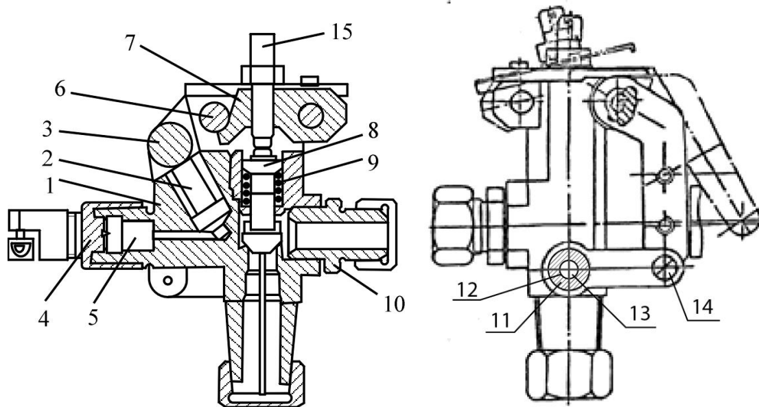
Рис. 3.11 – Запільно-пускова головка:
