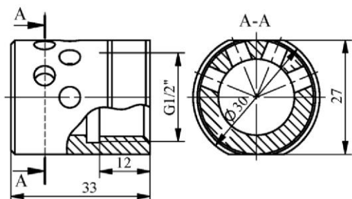
Рис. 2.10 – Насадок настінного типу з розпилом на 180^\circ для модуля типу «Імпульс-2-Т»
