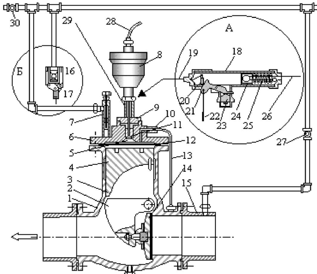
Рис. 1.20 – Клапан швидкодіючий з електромеханічним (КБГЭМ) і дублюючим гідравлічним приводами (КБГЭМ-М):
