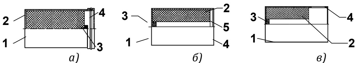
Рис. 4.7 – Варіанти типових схемних рішень ГВА серії АГС:
