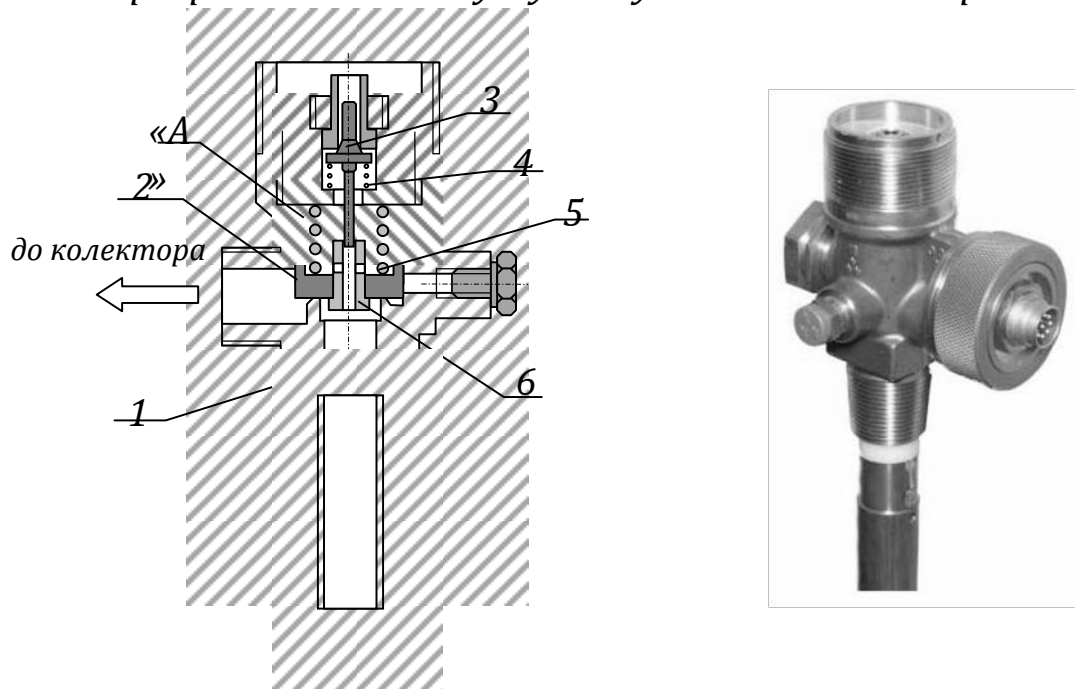
Рис. 2.4 – Головка запірня клапанного типу:
