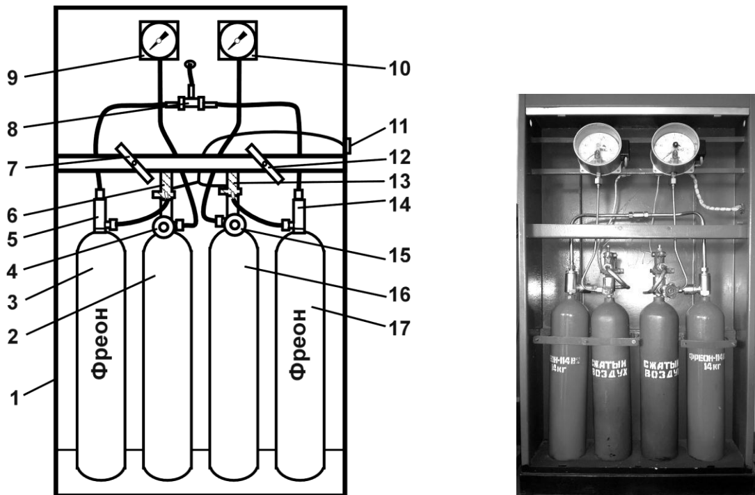
Рис 2.17 – Конструкція модульної установки:
