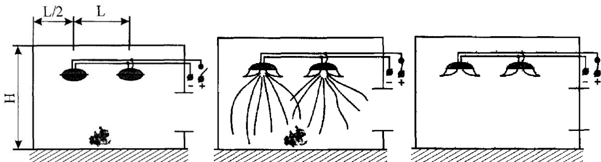
Рис.3.20 – Принцип роботи МПП «Буран»
