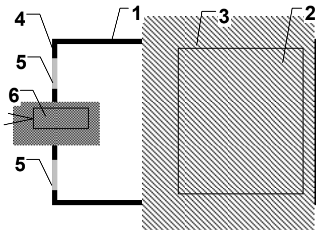
Рис. 4.2 – Принципова схема генератора вогнегасного аерозолу:
