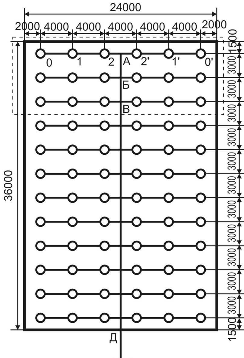
Рис. 1– Розрахункова схема спринклерної системи пожежогасіння
