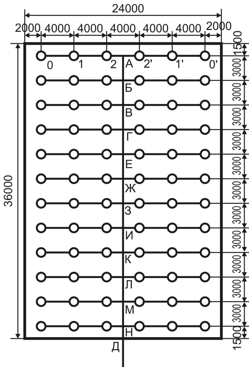
Рис. 2– Розрахункова схема дренчерної системи пожежогасіння
