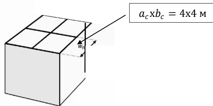
Рисунок 3.1 – Проектування блискавкоприймальної сітки
