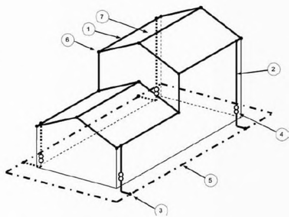
Рисунок 7.4 – Встановлення зовнішньої LPS на будівлі з різнорівневим дахом
