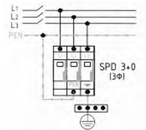
Рисунок 9.5 – Підключення ПЗІП класу II у системі TN-C
