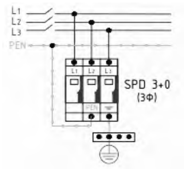
Рисунок 9.2 – Підключення ПЗП класу I у системі TN-C (TN-C-S).
