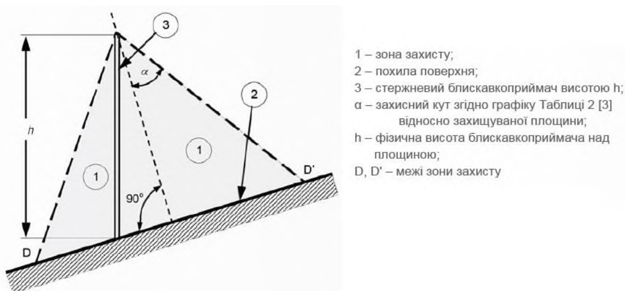
Рисунок 8.14 – Приклад захисту установок стрижневим блискавкоприймачем для похилої поверхні
