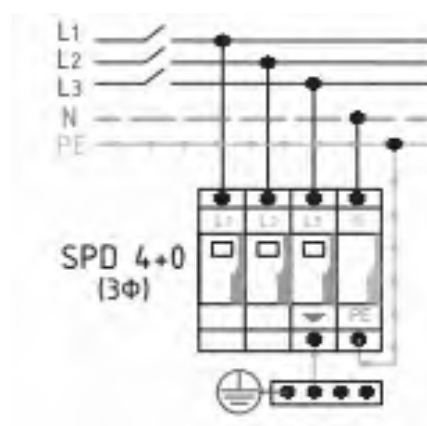
Рисунок 9.8 – Підключення ПЗІП класу II у системі TN-S (TN-C-S) у спосіб «х+1»
