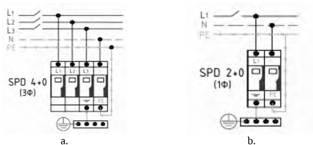
Рисунок 9.3 – Підключення ПЗП класу I у системі TN-S (TN-C-S): а – для 3-фазної мережі; б – для 1-фазної мережі.
