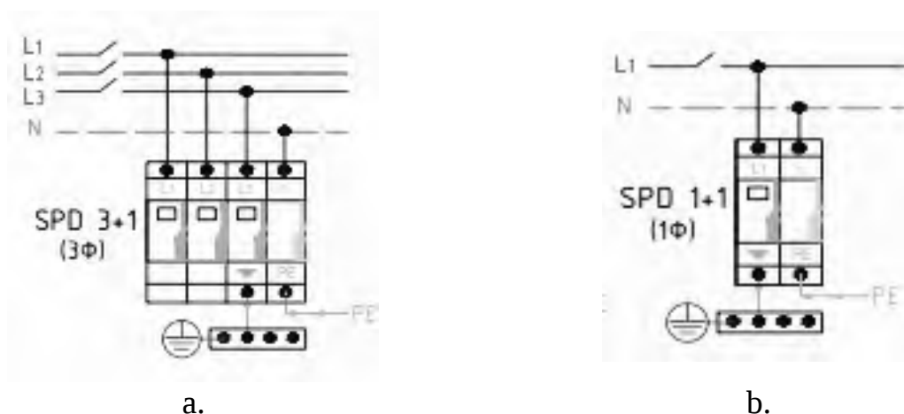
Рисунок 9.7 – Підключення ПЗІП класу II у системі TN-S (TN-C-S) у спосіб «х+0»: а – для 3-фазної 4-провідної мережі; б – для 1-фазної 2-провідної мережі.
