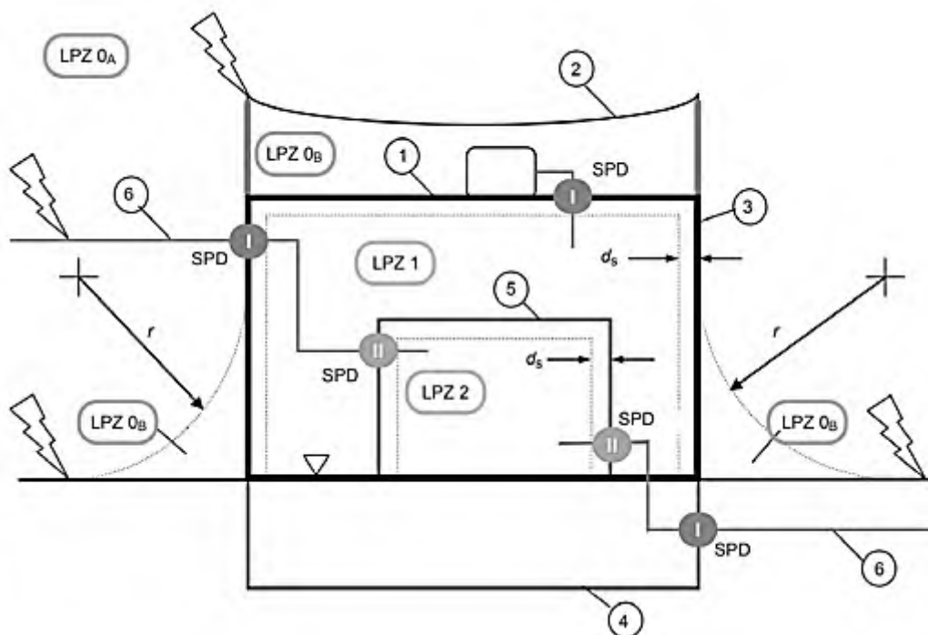
Рисунок 9.1 – Місця встановлення ПЗІП (SPD):
