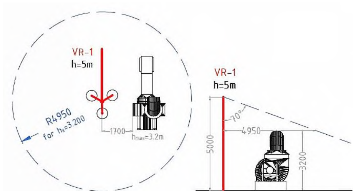
Рисунок 8.13 – Приклад захисту установок стрижневим блискавкоприймачем
