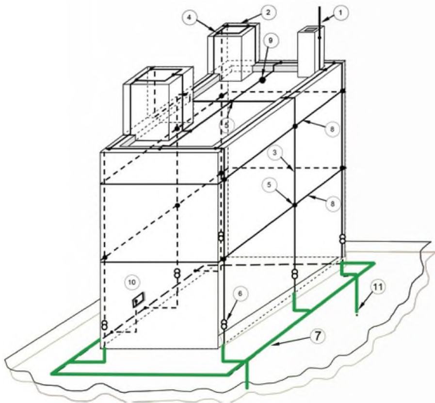
Рисунок 7.9 – Приклад LPS будівлі з розміщенням уземлення типу В
