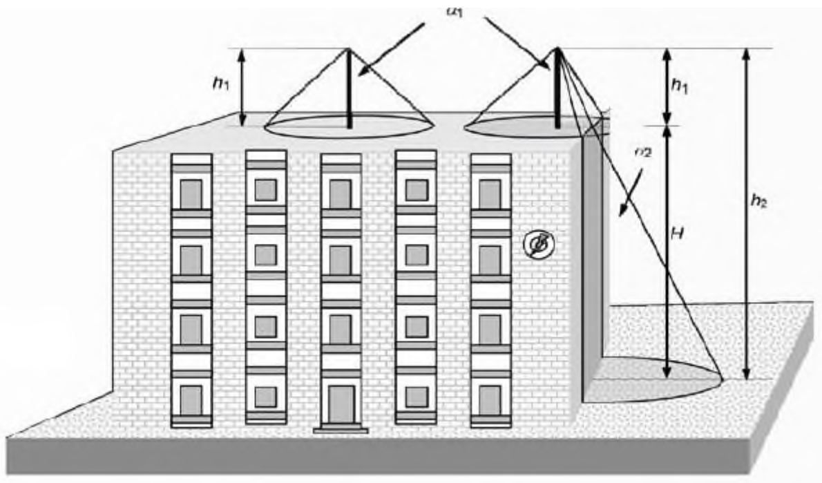
Рисунок 8.11 – Графічне відображення захисних кутів
