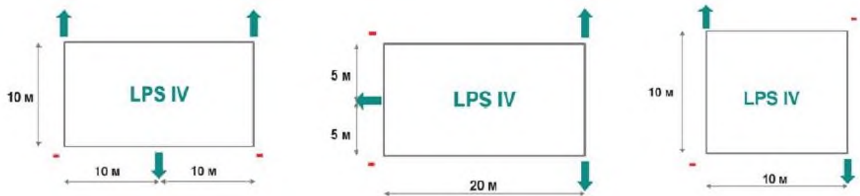
Рисунок 7.5 – Приклади будівель з LPS IV, для яких не потрібне встановлення струмовідводів у деяких виступаючих кутах
