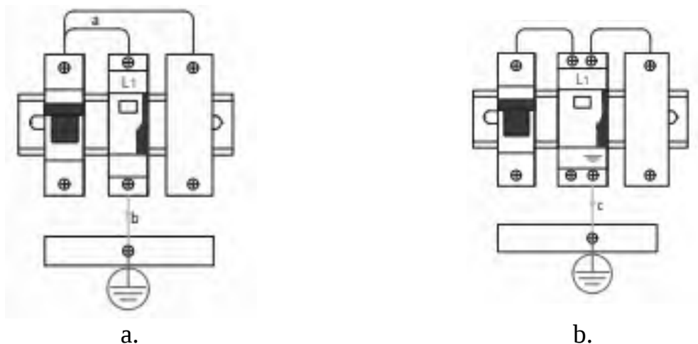
Рисунок 9.9 – Типи підключення ПЗІП: а – паралельне; б – послідовне
