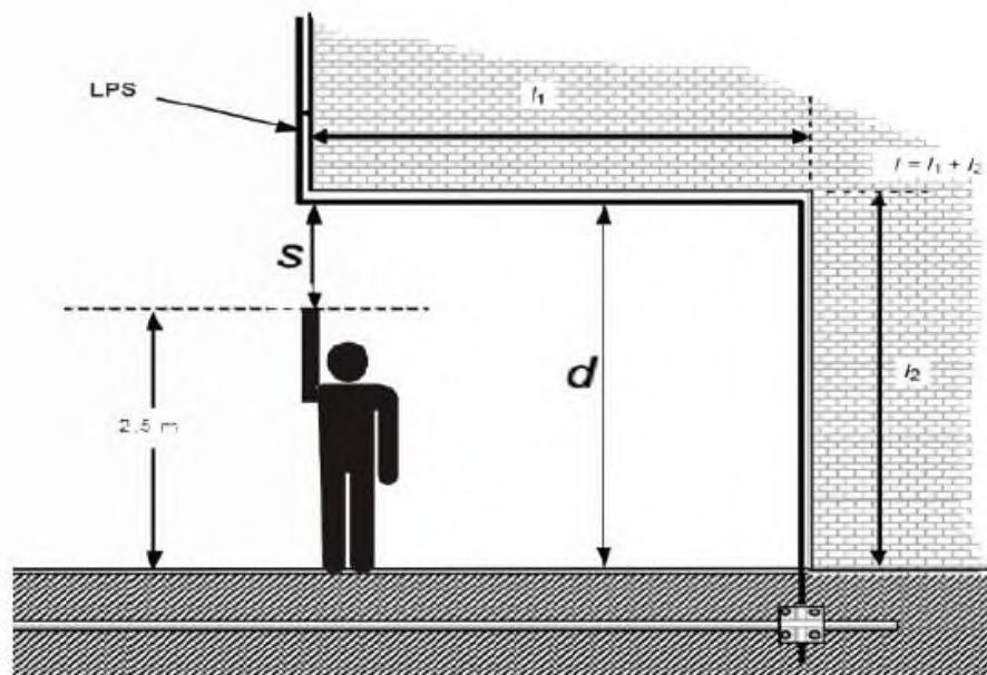
Рисунок 7.6 – Приклади будівель з LPS IV, для яких не потрібне встановлення струмовідводів у деяких виступаючих кутах
