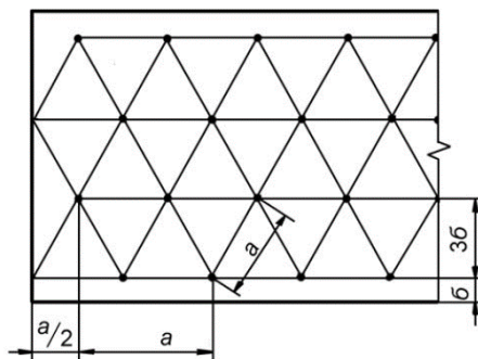
Рисунок 2.8.1.1. Схема трикутного розміщення сповіщувачів a – відстань між сповіщувачами; b – відстань від стіни до сповіщувача
