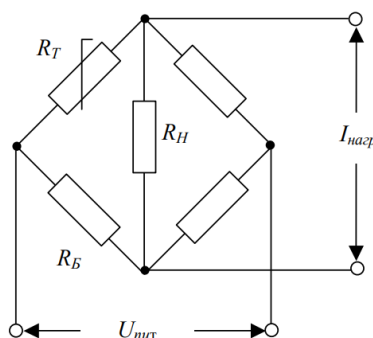
Рис. 2.2.3.2. Мостова схема підключення терморезистора
