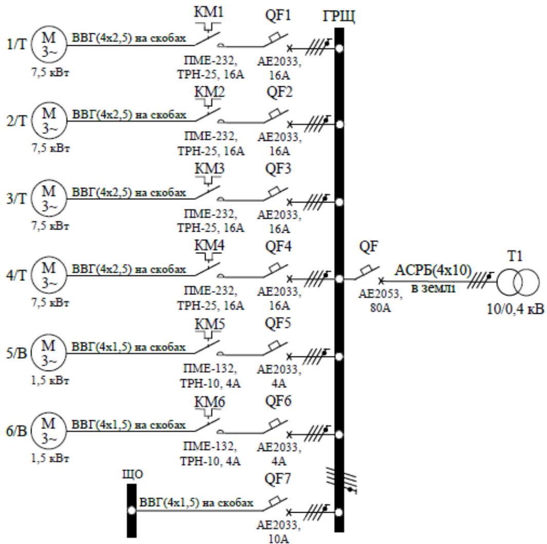
Рис. 3.1 – Розрахункова однолінійна схема електропостачання
