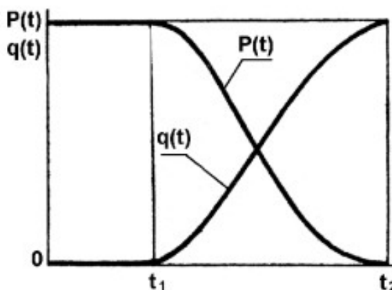
Рис. 1 – Залежність ймовірності безвідмовної роботи та ймовірності відмов від часу
