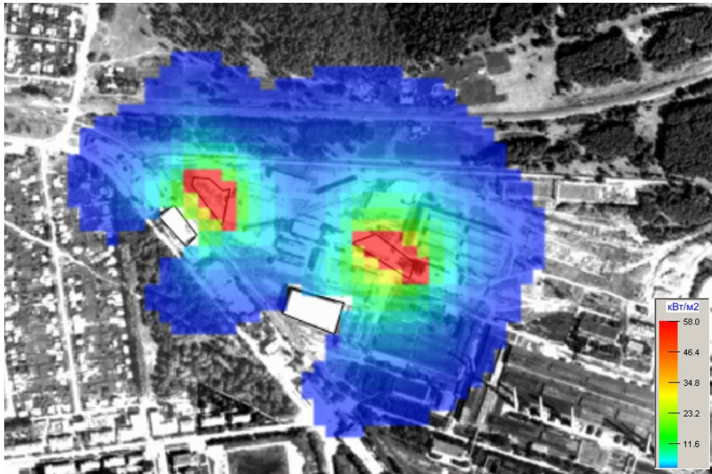
Рис. 2 – Зони впливу інтенсивності теплового випромінювання пожежі.
