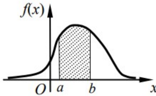
Рис. 2 – Крива диференціальної функції розподілу (щільність розподілу) випадкової величини X
