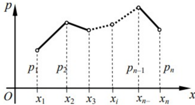
Рис. 1 – Багатокутник розподілу випадкової величини X
