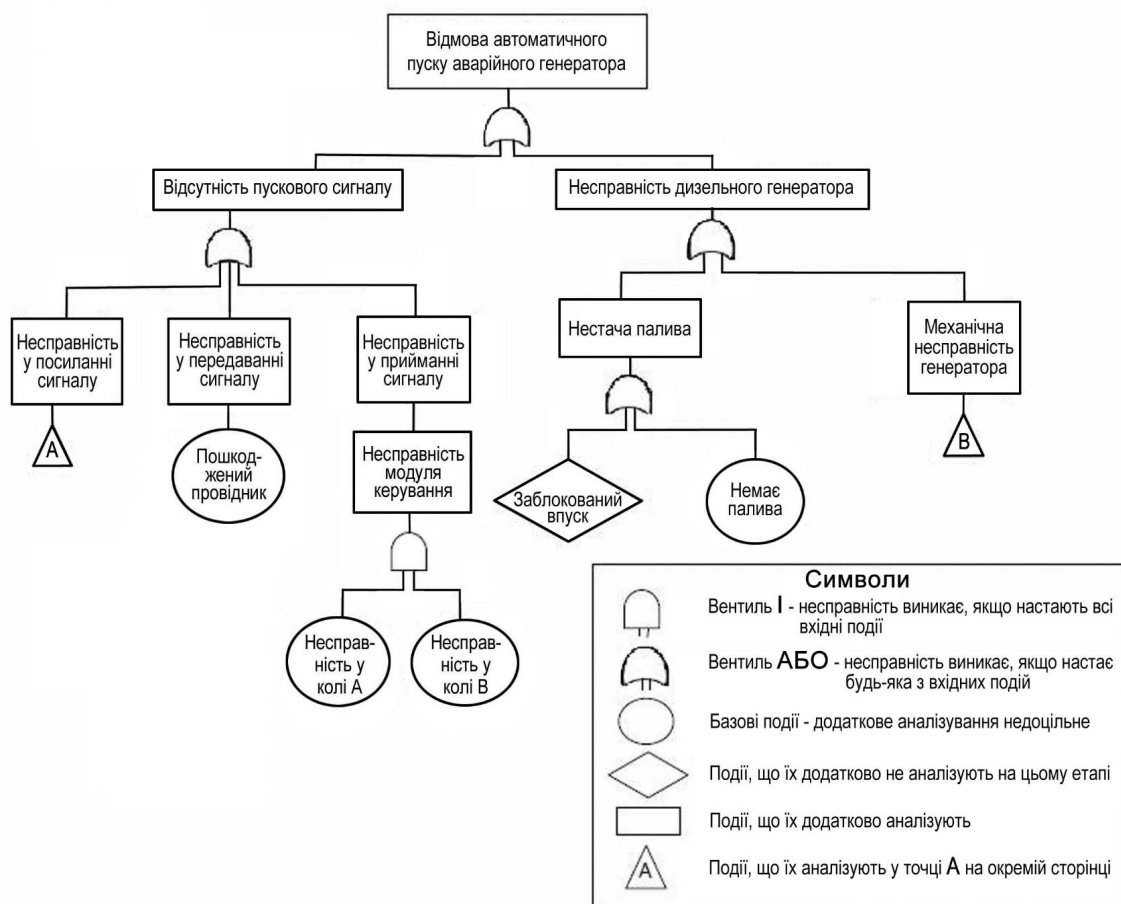
Рис. 1 – Приклад дерева відмов
