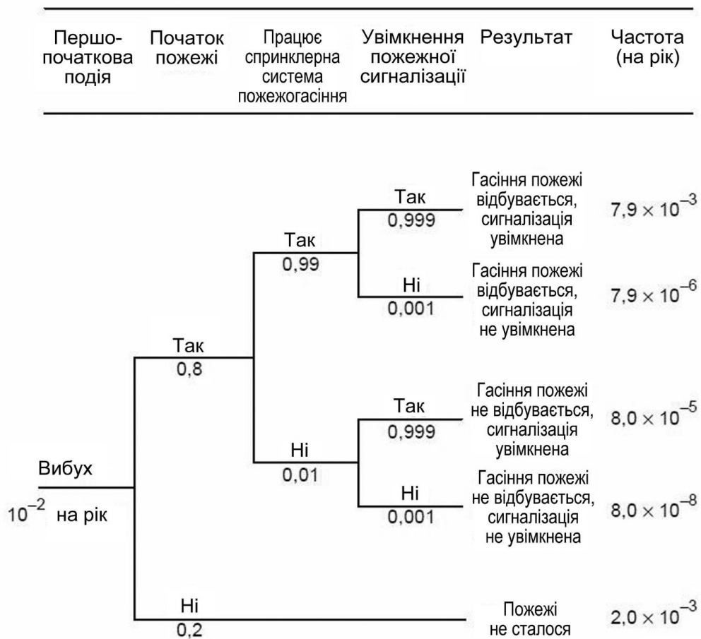
Рис. 2 – Приклад дерева подій
