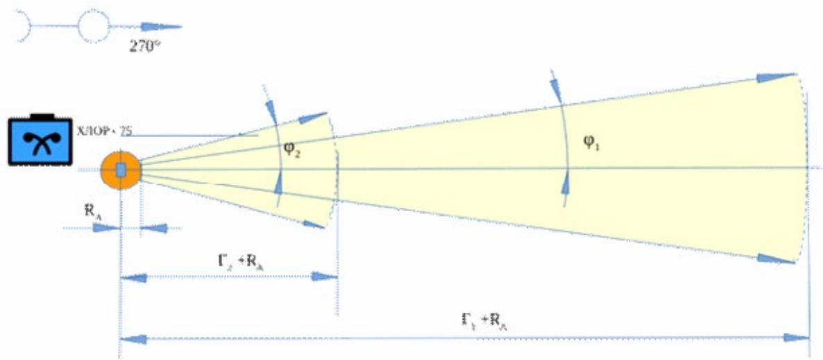
Рис. 1 – Схема поширення первинної та вторинної хмари НХР
