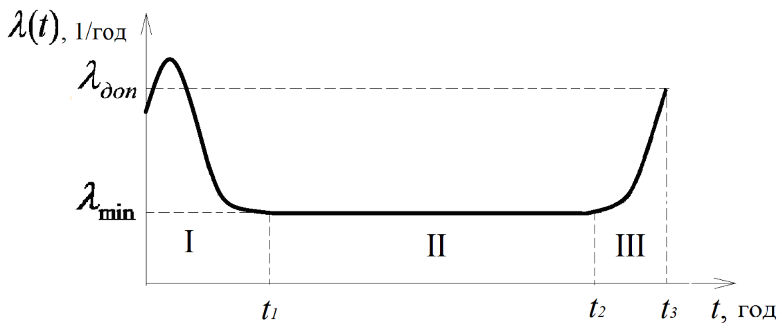
Рисунок 2 – Залежність інтенсивності відмов від часу
