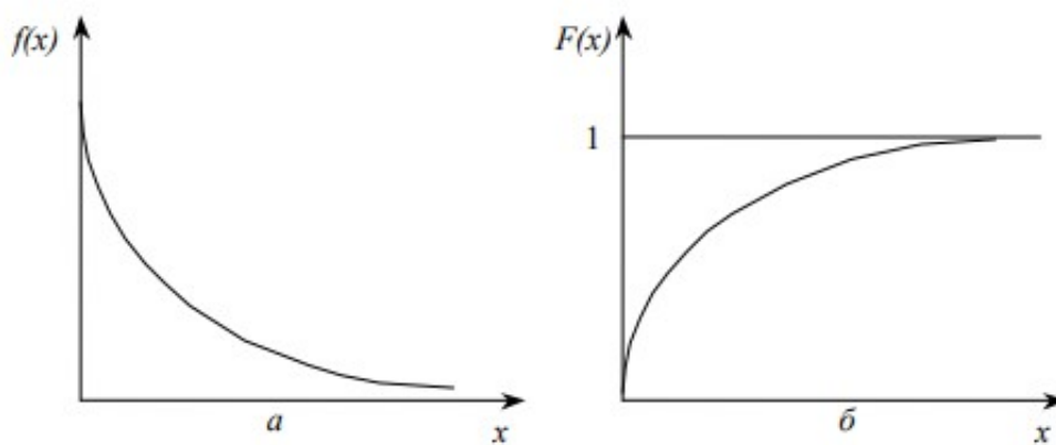
Рис. 5. Диференціальна (а) та інтегральна (б) функції показникового розподілу.
