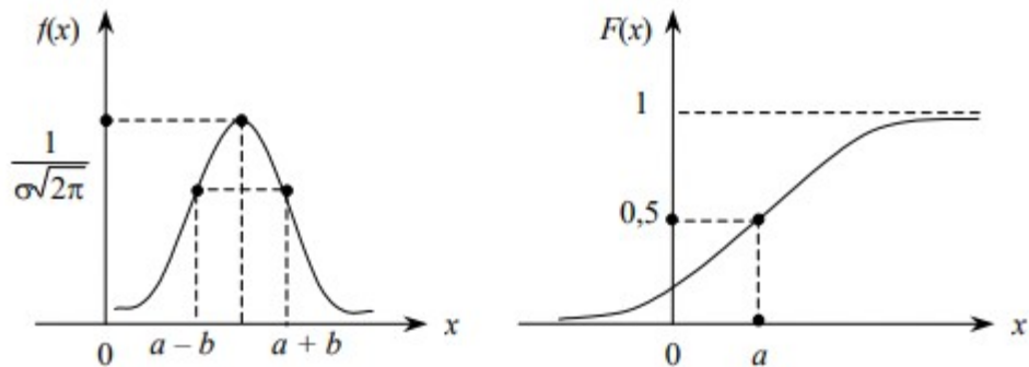
Рис. 4 – Щільність розподілу ймовірностей (диференціальна функція розподілу випадкової величини) (а) і функції розподілу (б) для нормального розподілу
