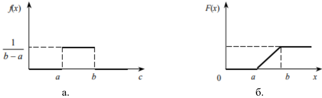
Рис. 3 – Щільність розподілу ймовірності (диференціальна функція розподілу випадкової величини) (а) і функції розподілу (б) для рівномірного розподілу
